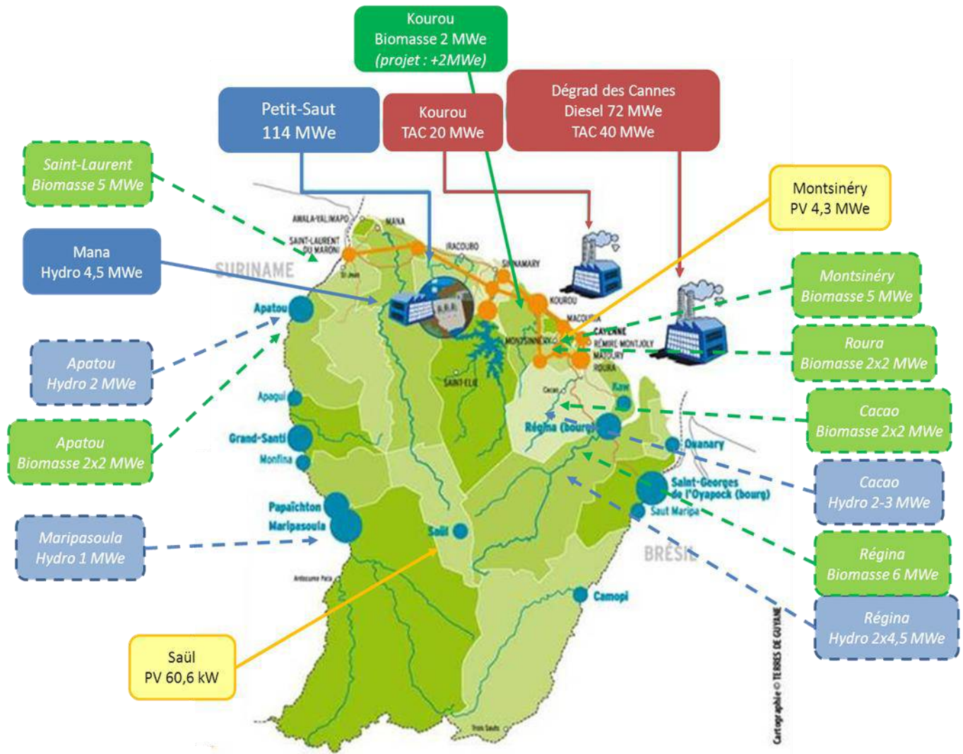
Carte du système électrique existant et des projets énergies renouvelables en Guyane
